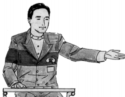
3.4.1.1.2 "Nouveau serveur"
