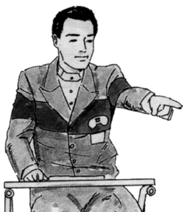
3.4.1.6 "Côté"
